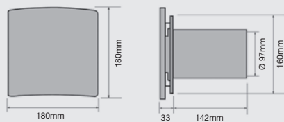
Wall fan
