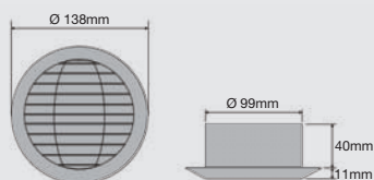
Ceiling fan
